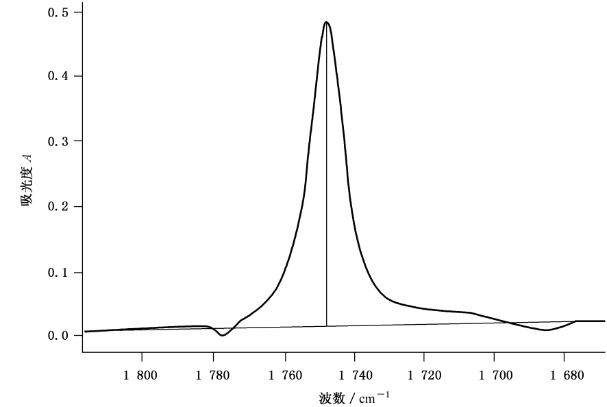
图 1 用环己烷稀释后的柴油机燃料中 FAME 的典型红外光谱图 (样品池 0.5 mm, 将 FAME 质量浓度为 44 g/L 的试样按体积比 1 : 10 稀释)
